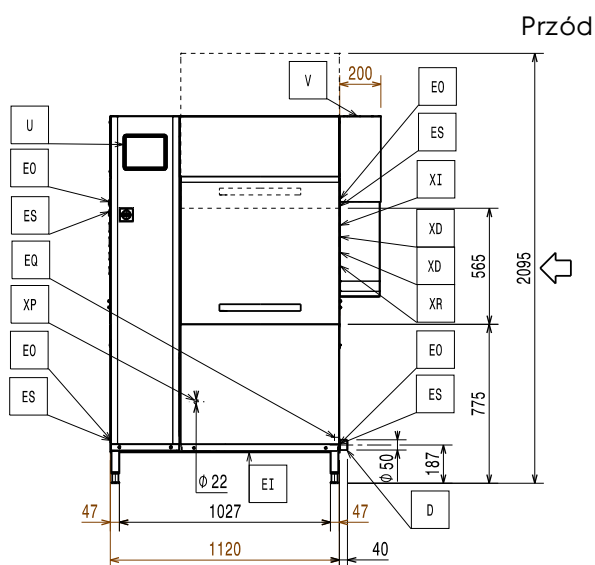
Bok
