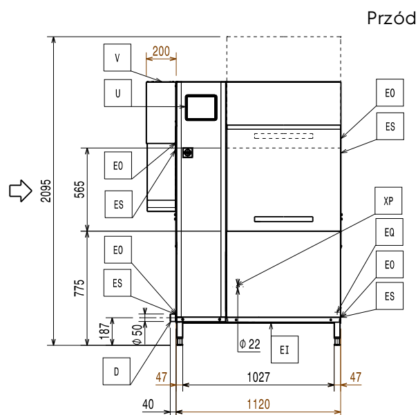
Bok
